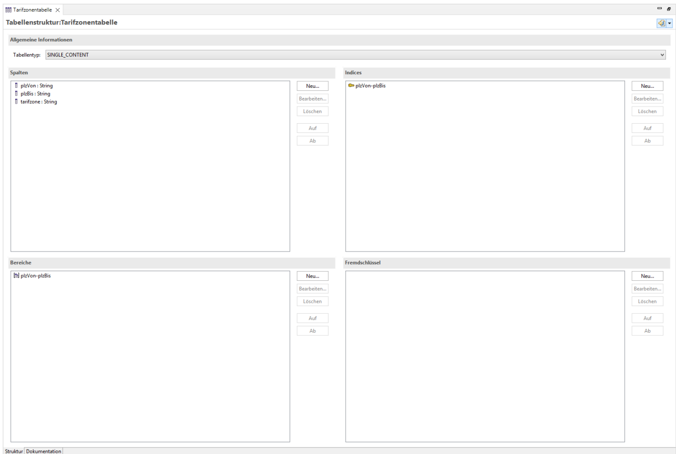
Figure 69. Tabellenstruktur Tarifzontabelle
