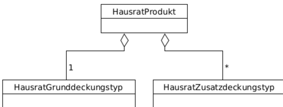
Figure 25. Modell der Produktkonfigurationsklassen
