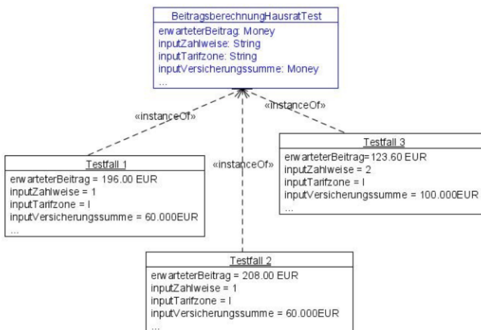
Figure 97. Testfälle als Instanzen vom Testfalltyp BeitragsberechnungHausratTests
