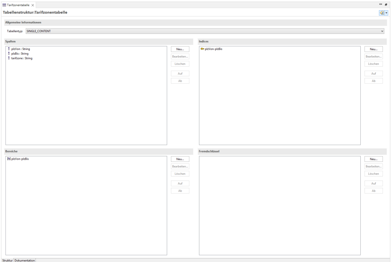
Figure 67. Tabellenstruktur Tarifzontabelle
