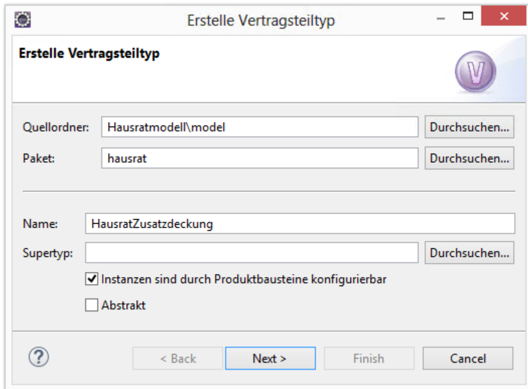
Figure 76. Assistent zum Anlegen der Vertragsklasse HausratZusatzdeckung
