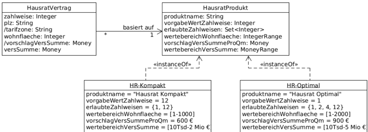
Figure 18. Hausratmodell mit Produktklassen
