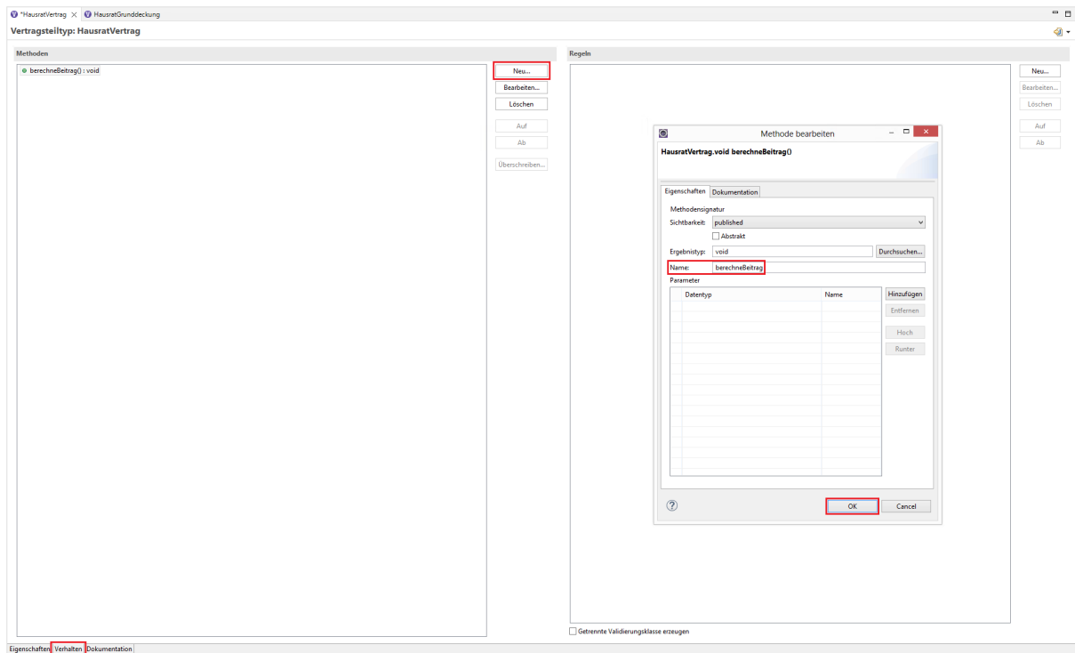
Figure 72. Dialog zum Bearbeiten einer Methodensignatur
