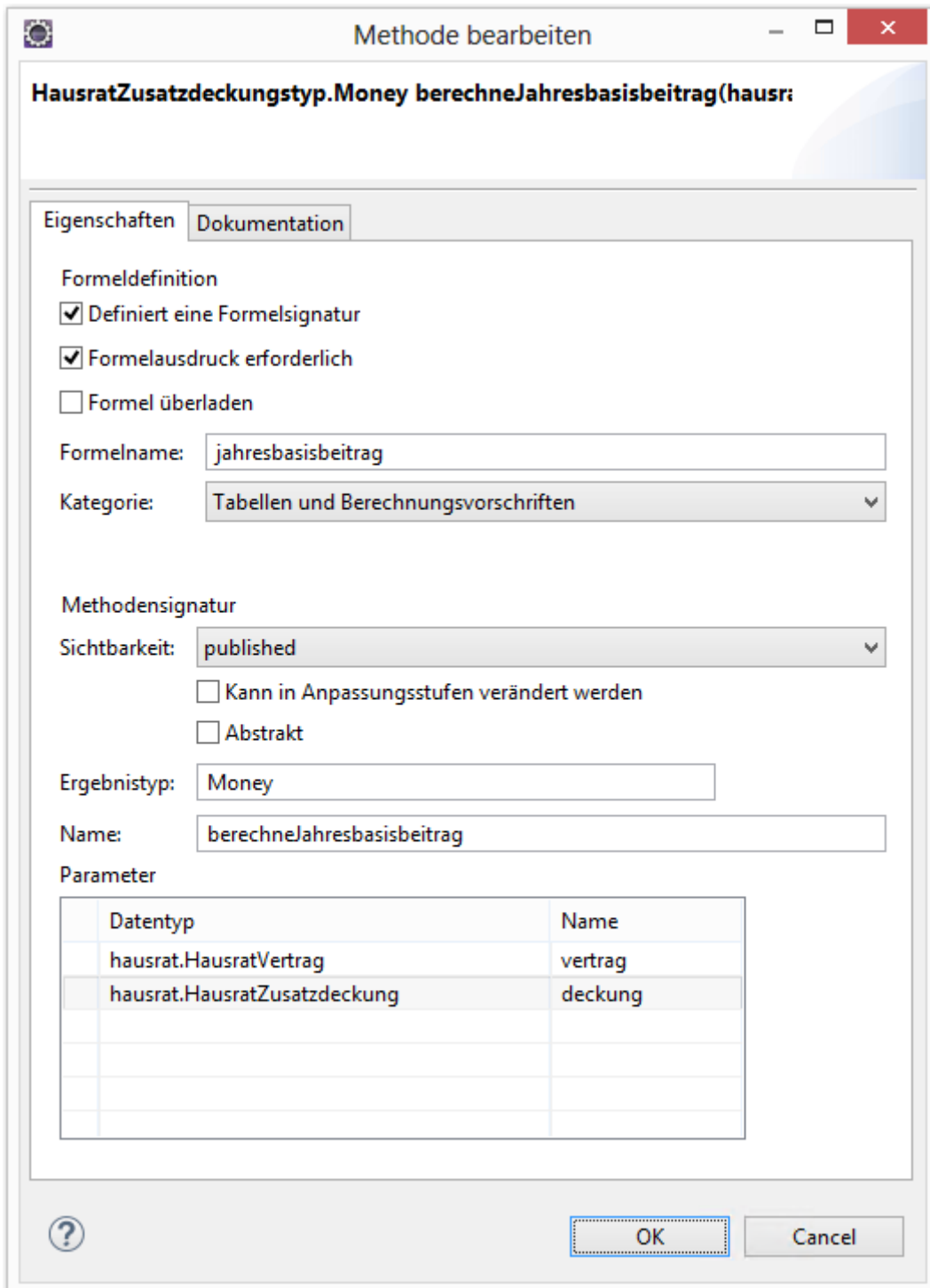
Figure 78. Dialog zur Definition einer Formelsignatur
