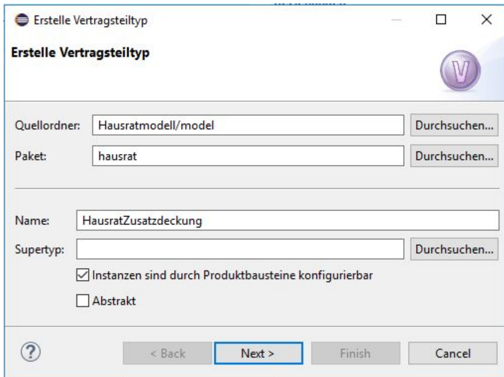
Figure 46. Assistent zum Anlegen der Vertragsklasse HausratZusatzdeckung
