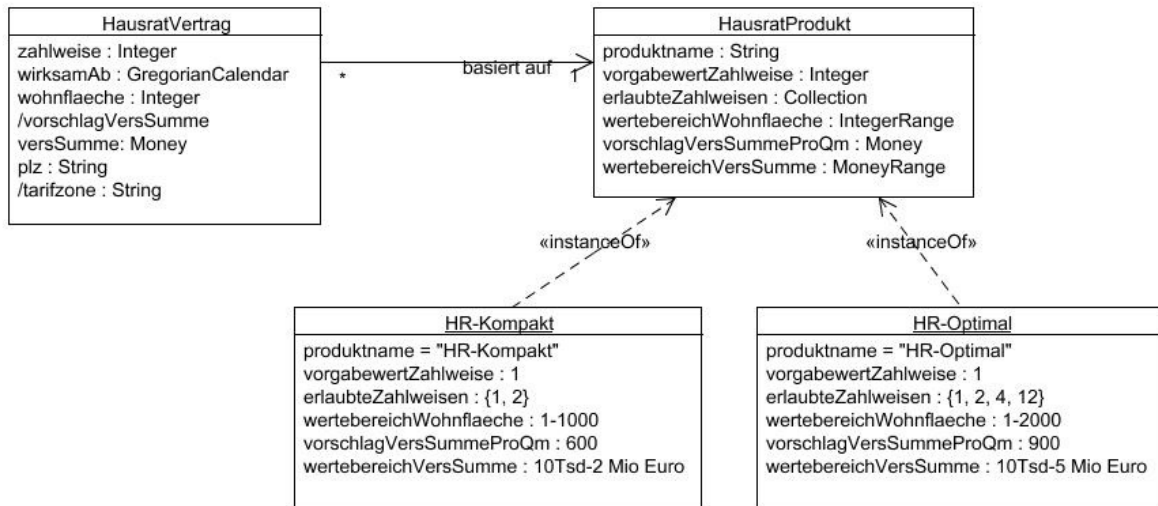
Figure 18. Hausratmodell mit Produktklassen
