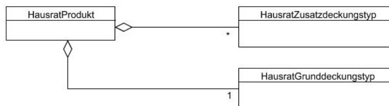
Figure 24. Modell der Produktkonfigurationsklassen
