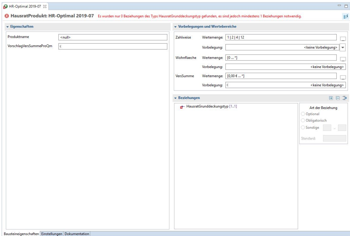
Figure 30. Produktbaustein-Editor für HR-Optimal
