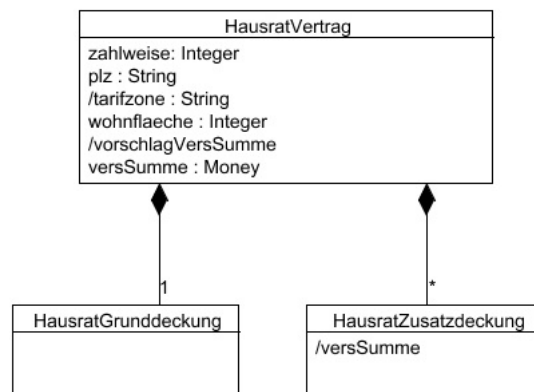
Figure 16. Hausratmodell mit Grunddeckung und Zusatzdeckung
