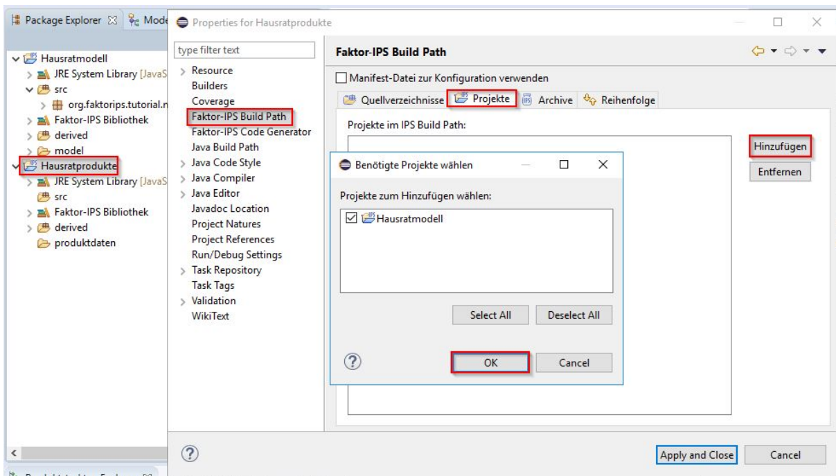
Figure 26. Referenz auf das Modell anlegen
