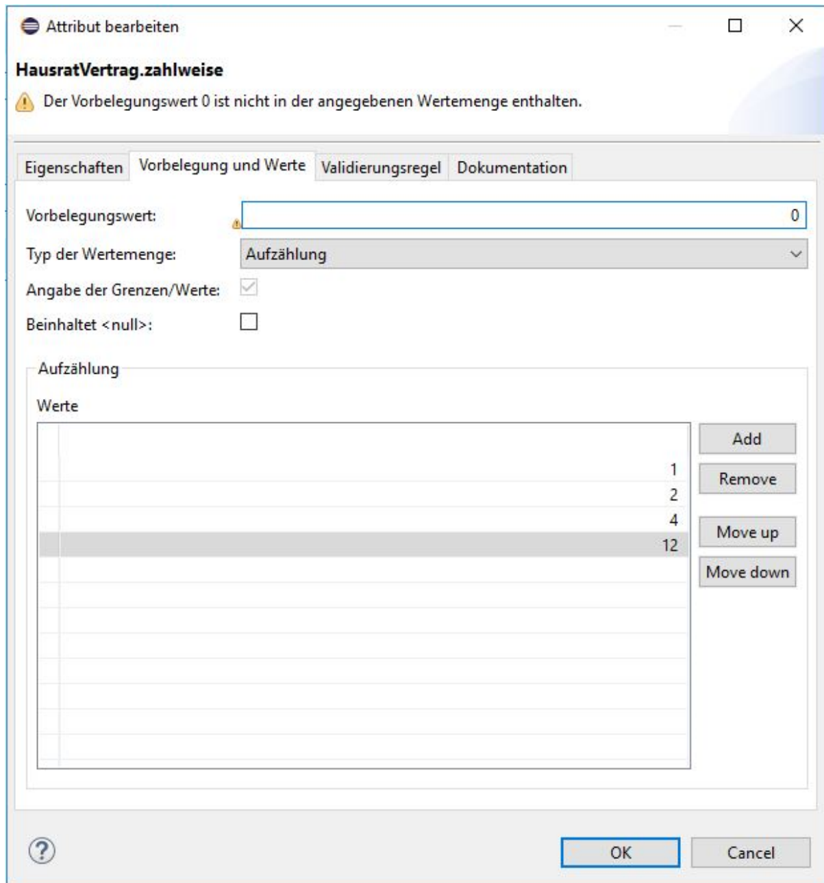
Figure 9. Wertebereich für das Attribut zahlweise
