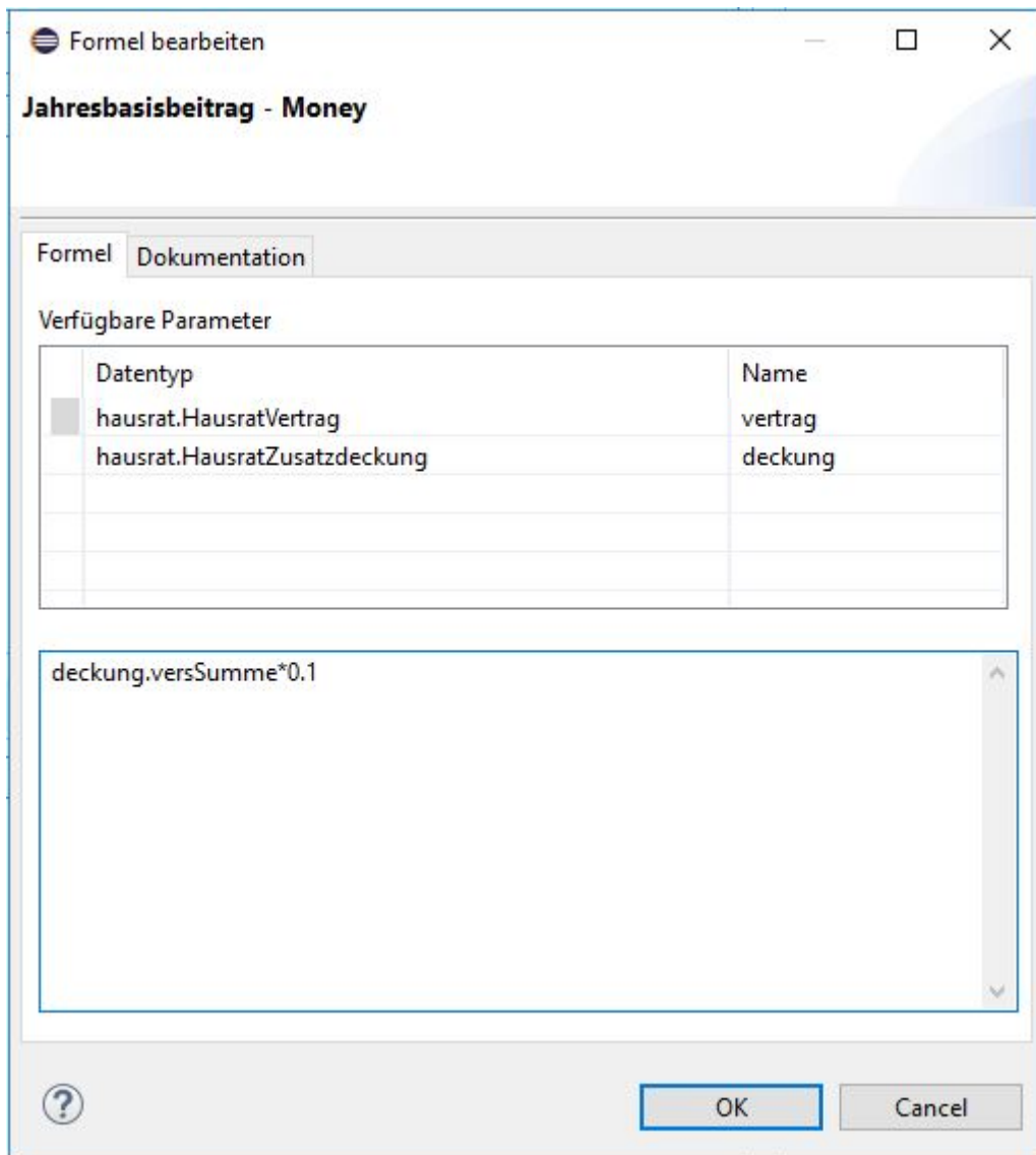
Figure 50. Anlegen einer Formel
