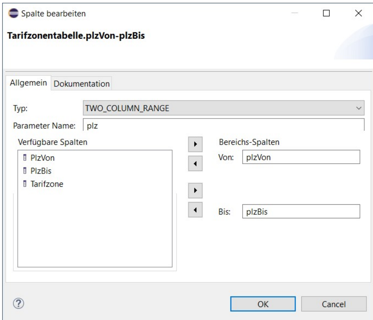
Figure 35. Bereich der Tabellenstruktur anlegen
