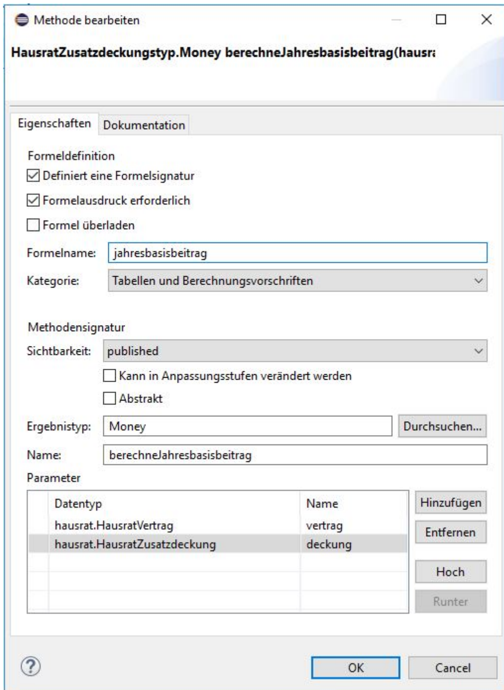
Figure 48. Dialog zur Definition einer Formelsignatur
