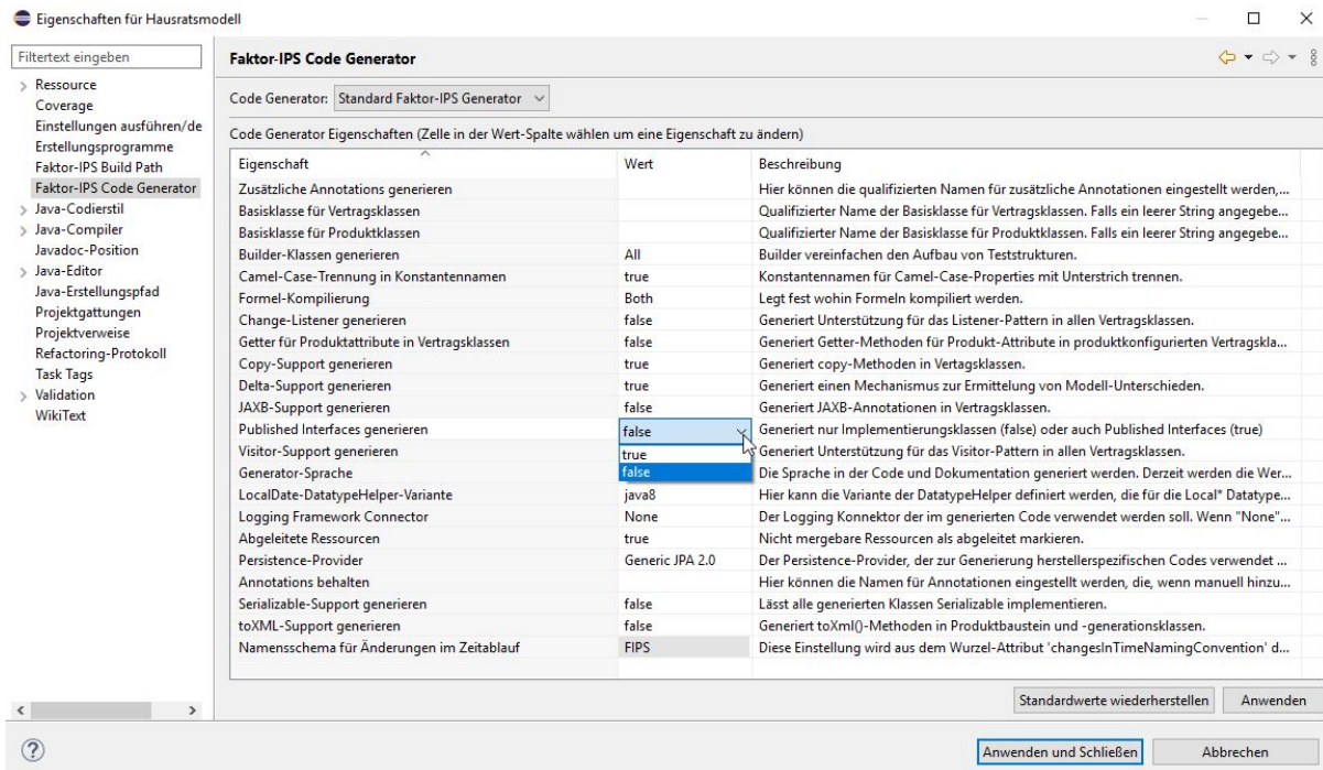
Figure 8. Aktivierung/Deaktivierung der Generierung der Published-Interfaces
