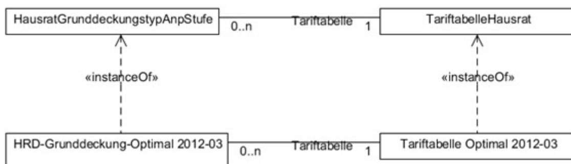
Figure 38. Zusammenhang Produktbausteine & Tabellen
