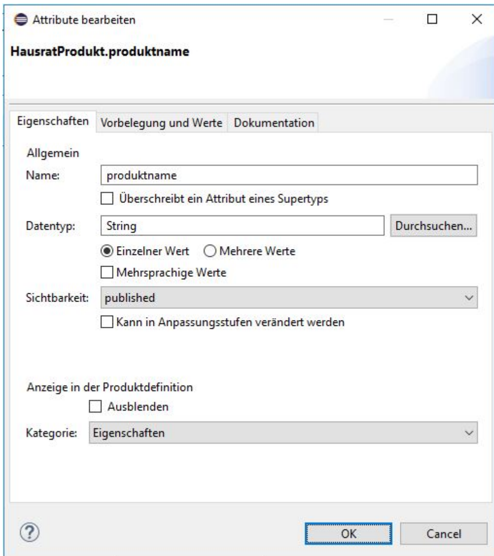
Figure 20. Dialog zum Editieren von Produktattributen
