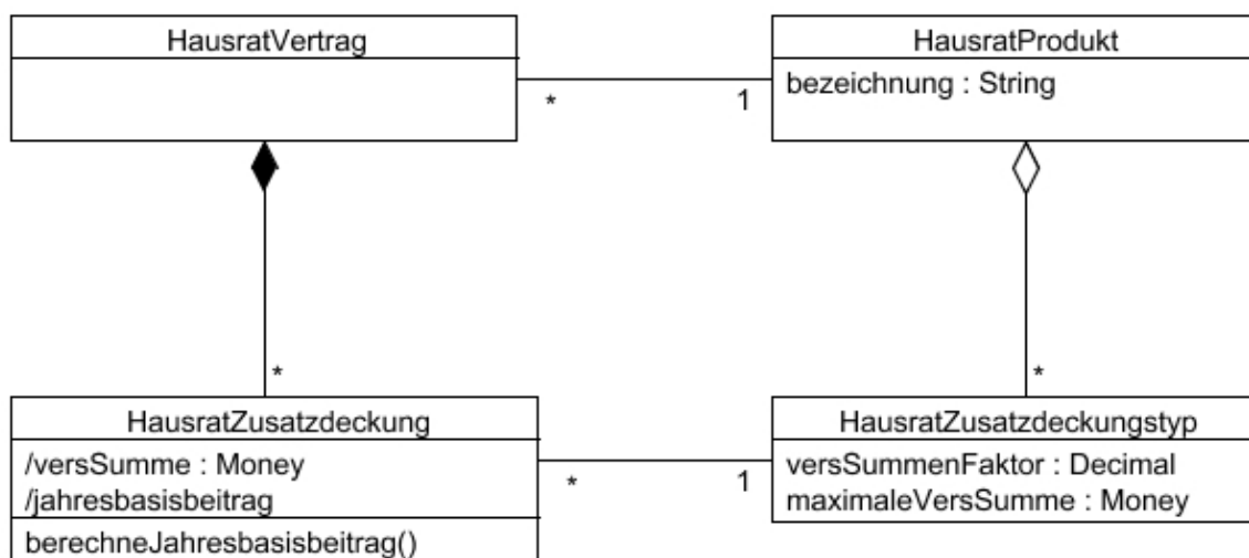
Figure 44. Modellausschnitt für Zusatzdeckungen
