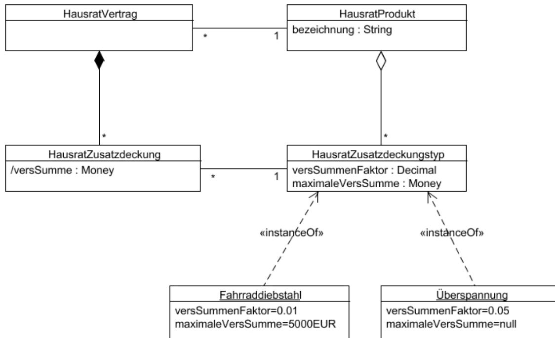
Figure 45. Modellausschnitt für Zusatzdeckungen mit Instanzen
