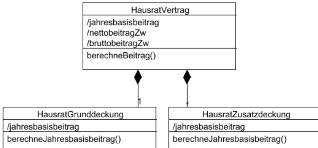
Figure 41. Berücksichtigung der Beitragsberechnung im Modell
