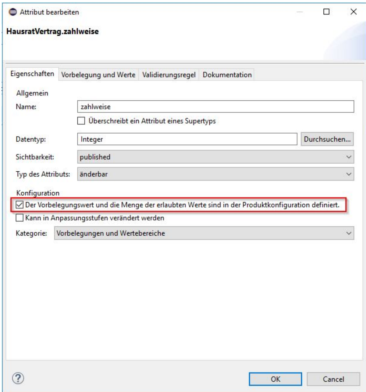
Figure 22. Dialog für ein Vertragsklassenattribut mit Konfigurationsmöglichkeit
