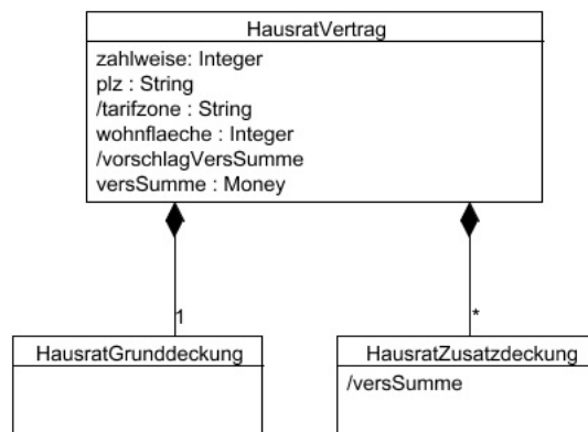
Figure 17. Hausratmodell mit Grunddeckung und Zusatzdeckung
