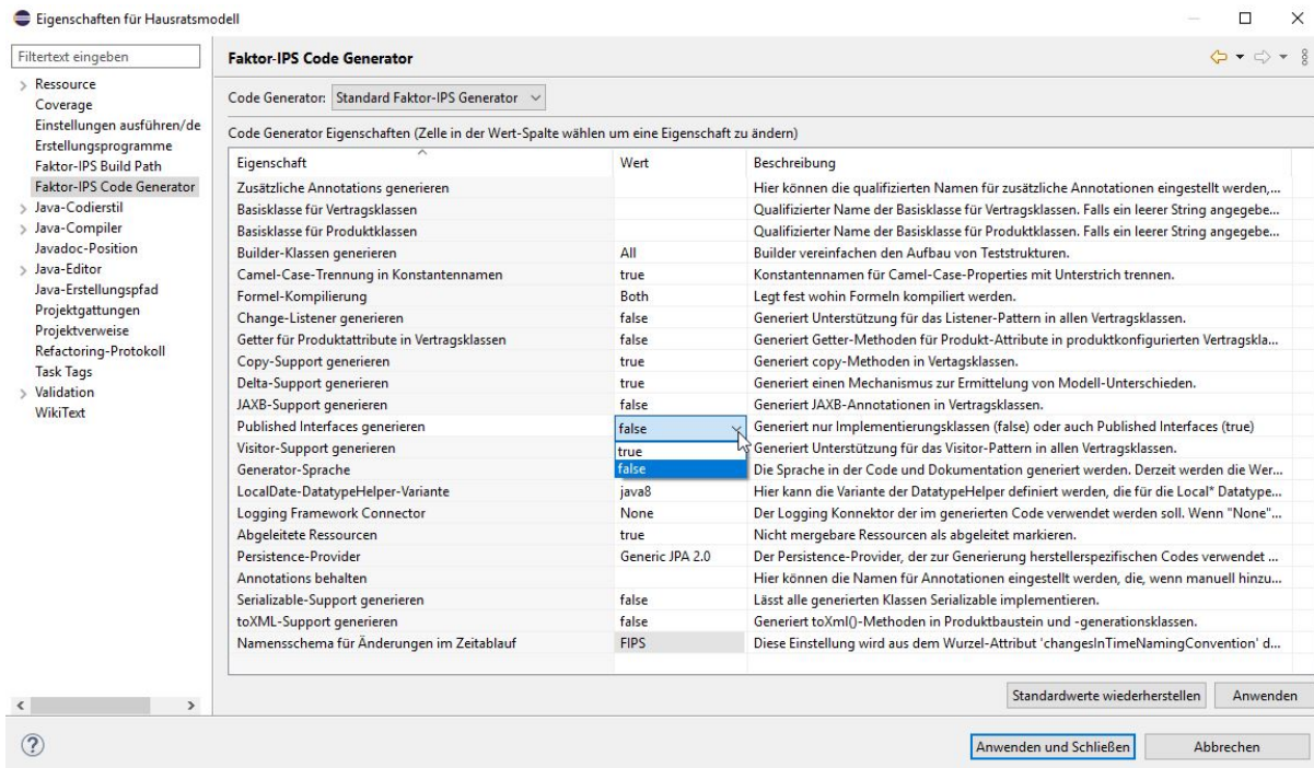
Figure 9. Aktivierung/Deaktivierung der Generierung der Published-Interfaces
