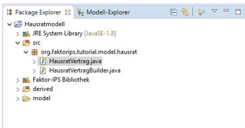
Figure 7. Generierte Klassen
